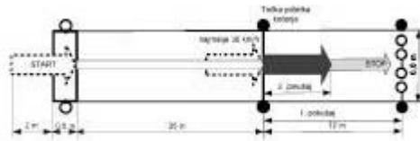
Slika 4. Prometno-tehnički element za kočenje i zaustavljanje vozila A1, A2, A i AM kategorije
