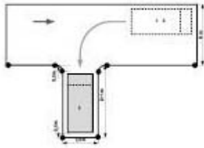
Slika 15. Prometno-tehnički element za parkiranje vozila C1 i C kategorije
