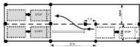
Slika 14. Prometno-tehnički element za vožnju unaprijed-unatrag s promjenom smjera za vozila C1E i CE kategorije
